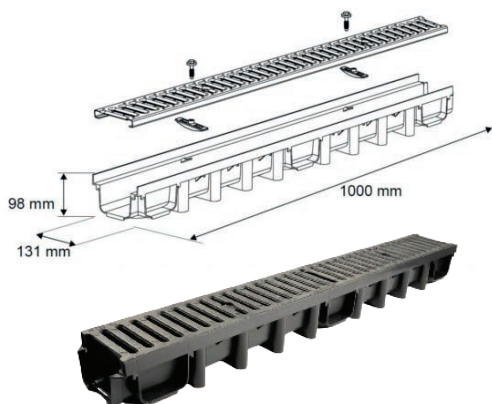
Odwodnienie z kratą żeliwną B125 lub C 250 wytrzymałość 12,5 tony lub 40 ton
